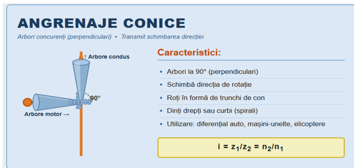
Fig. 2 – Angrenaj conic: transmite mișcarea cu schimbarea direcției de 90° (ex: diferențial auto).
