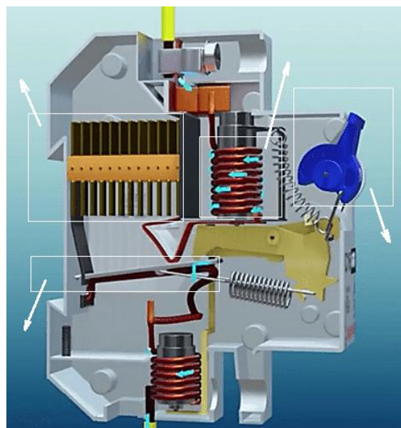
Întreruptor automat (secțiune)
