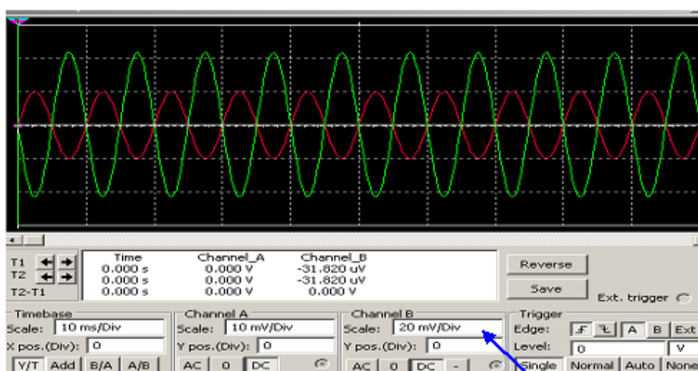
Fig. 3 Oscilograma fără condensatorul de decuplare C5 în schemă
