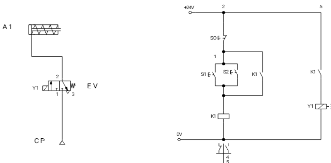
Comanda unui cilindru cu simplu efect
