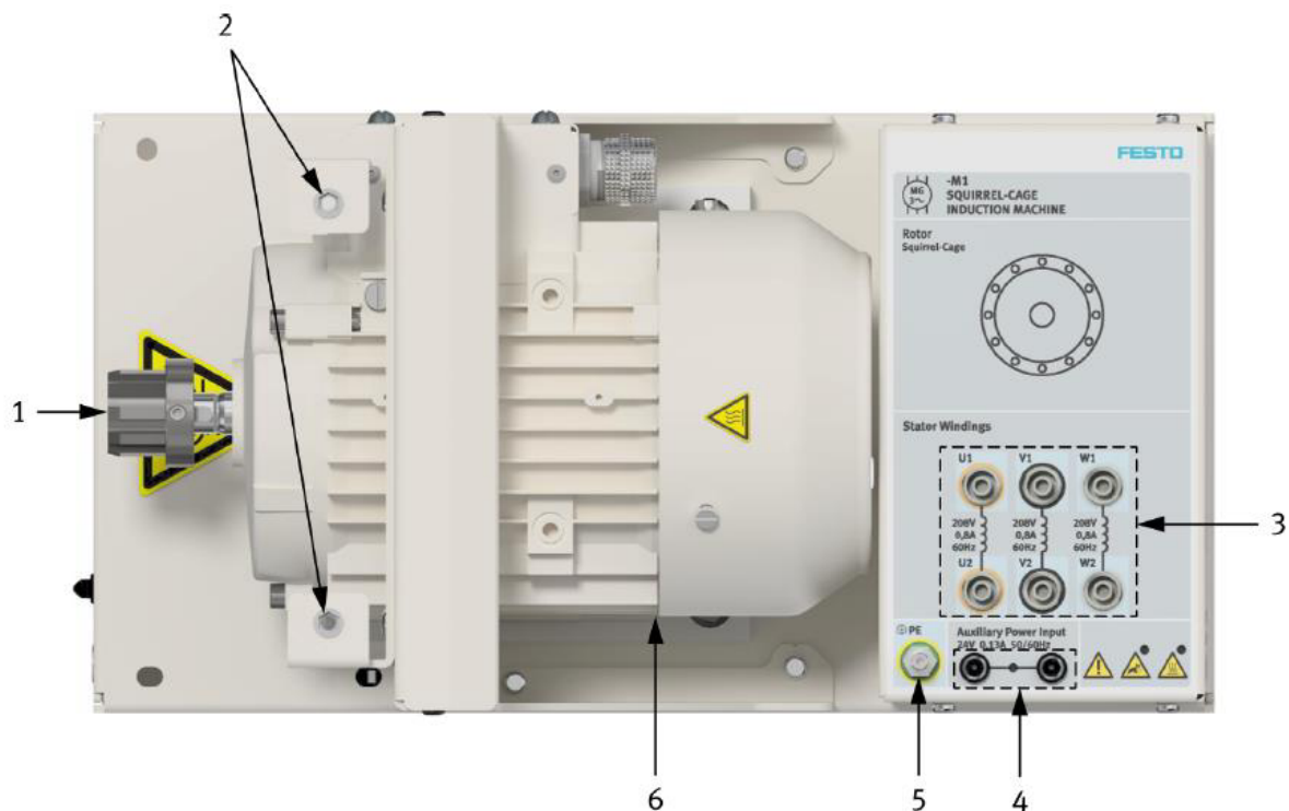
Figura. Motor asincron cu rotorul în colivie (Motor cu inducție cu colivie - Squirrel cage induction motor) (Ghid Festo Didactic - https://www.festo.com/ro )
