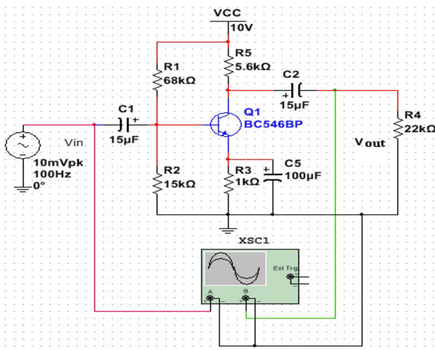
Fig. 1 Amplificator cu tranzistor bipolar în conexiunea emitor comun
