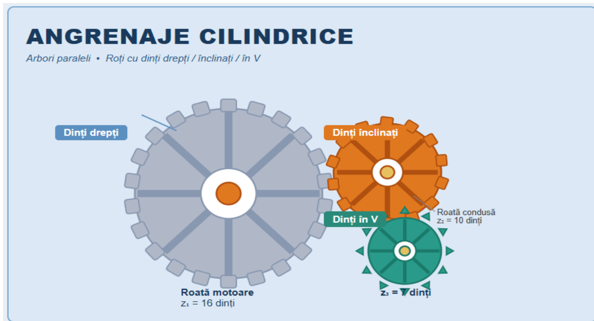
Fig. 1 – Angrenaje cilindrice: roată mare ( z=16 ) antrenează roata mică ( z=7 ) → turație dublă.
