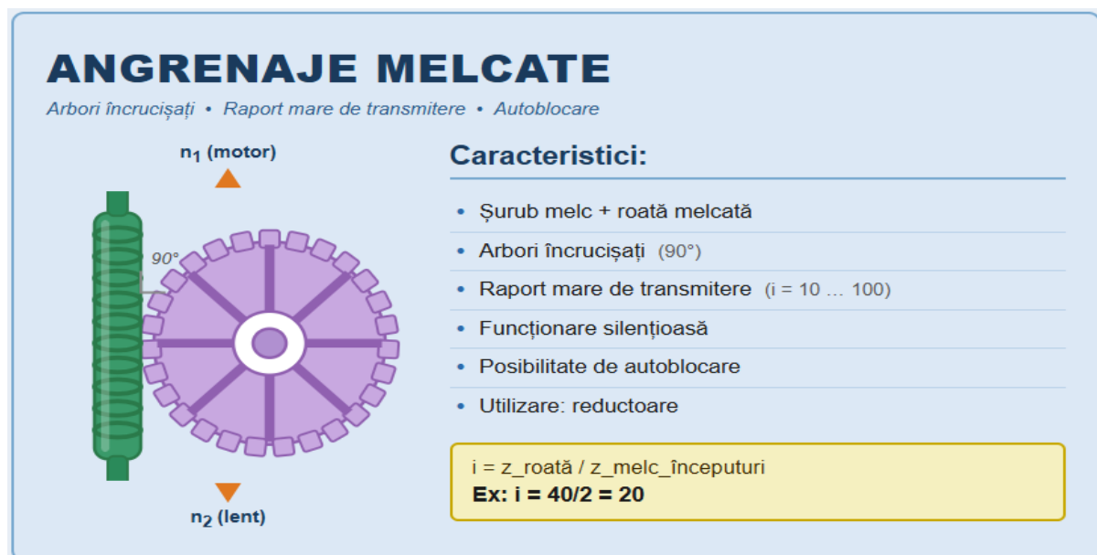
Fig. 3 – Angrenaj melcat: raport de transmitere i = 10\text{--}100 , funcționare silențioasă.
