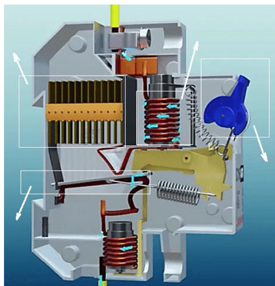
Întreruptor automat (secțiune)
