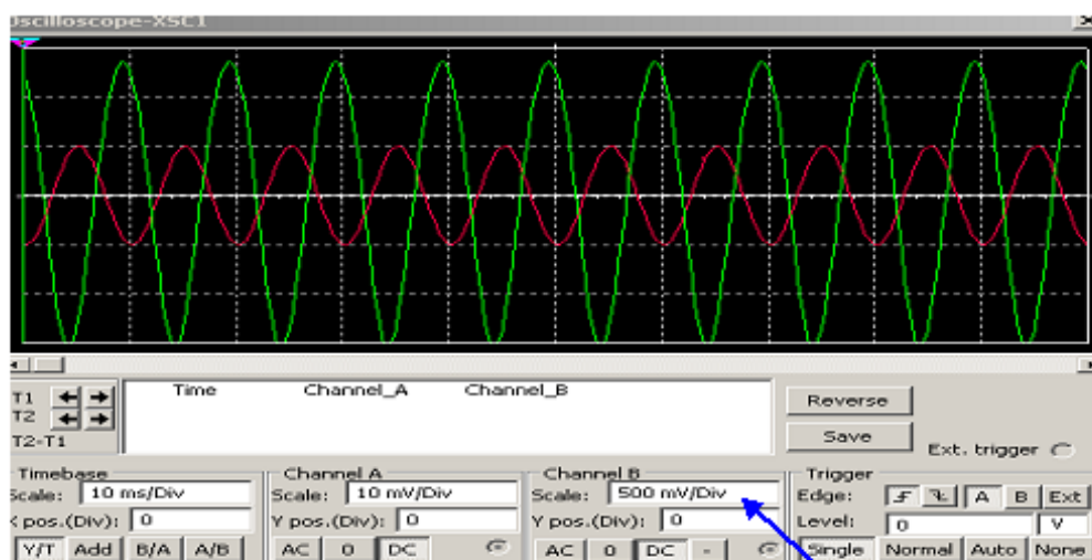
Fig. 2 Oscilograma cu condensatorul de decuplare C5 în schemă
