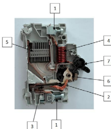
Fig. b Vedere în secțiune
