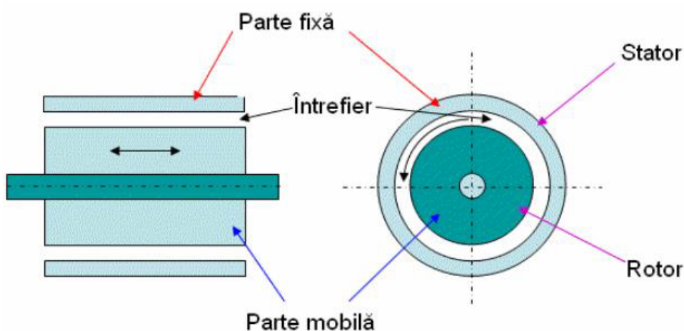
Figura. Elementele componente de bază ale mașinilor electrice:
